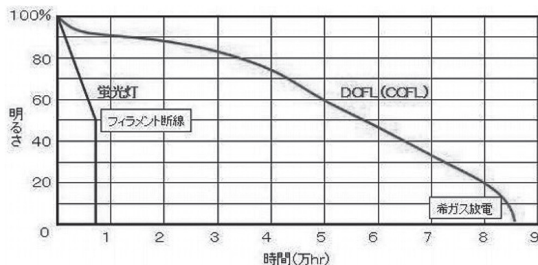
図5 寿命曲線
