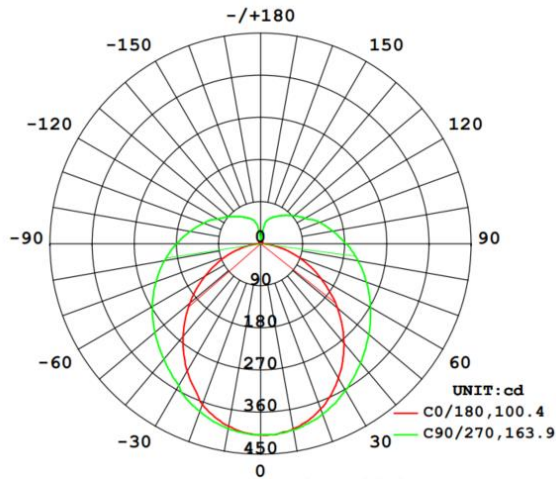
配光曲線および照度図
