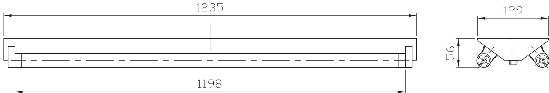
LEDランプ外形寸法
