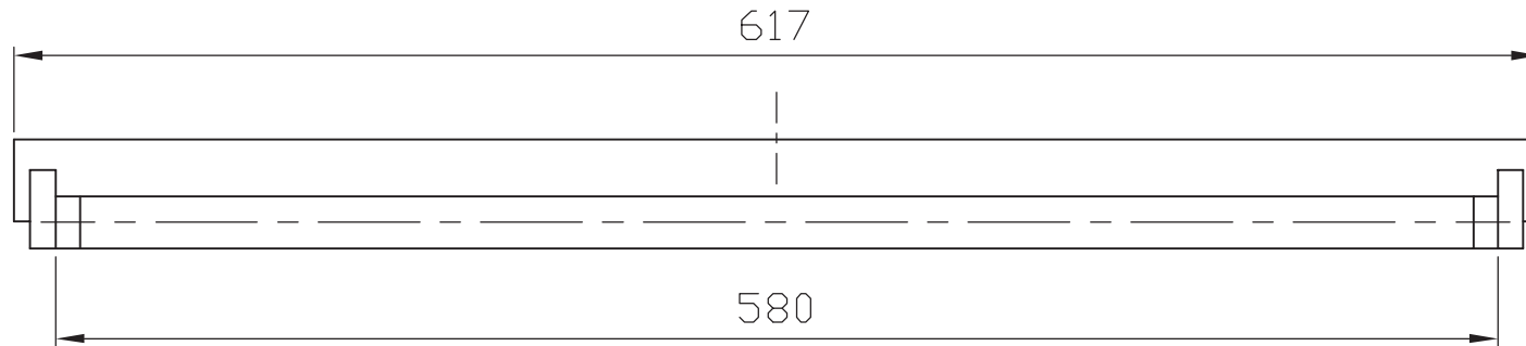
LEDランプ外形寸法
