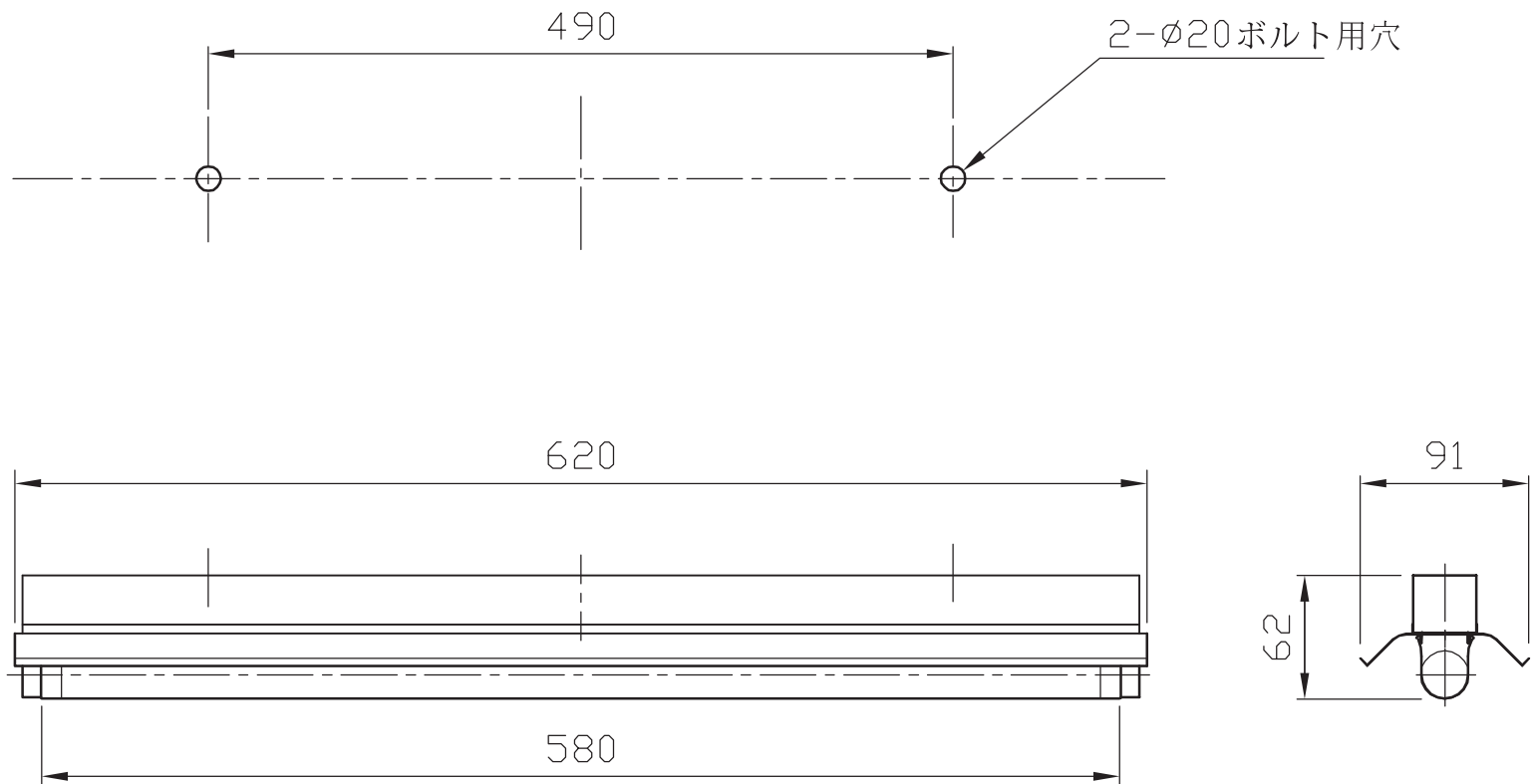
LEDランプ外形寸法
